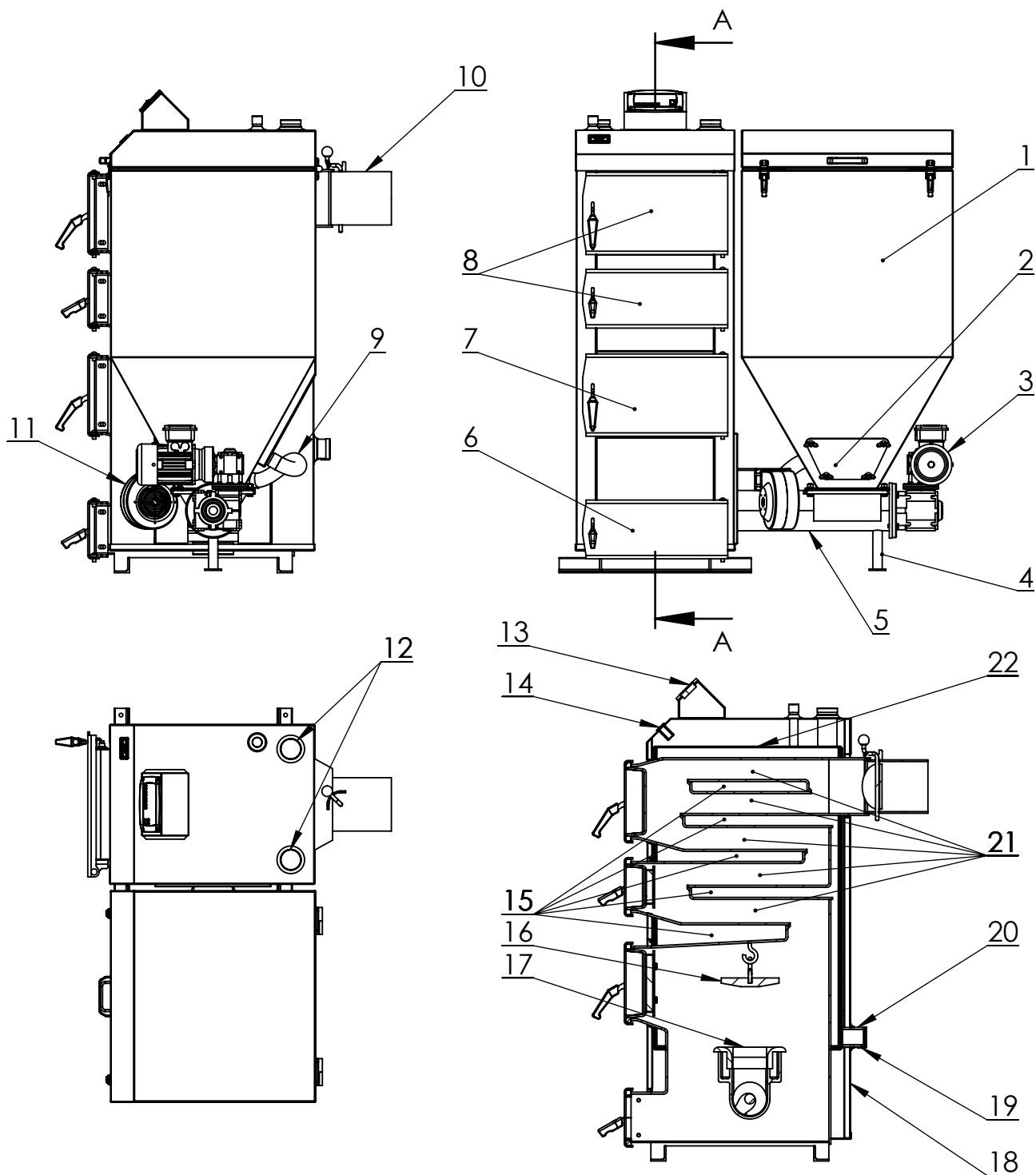
PRZEKRÓJ A-A
