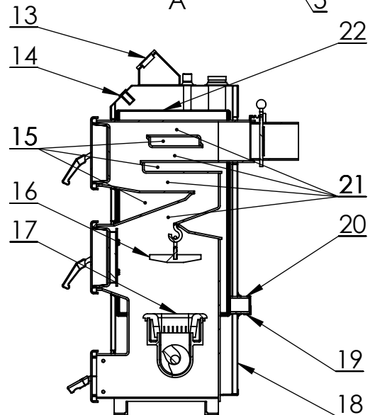
PRZEKRÓJ A-A
