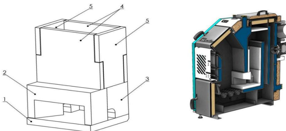
RYS. 3 PRAWIDŁOWE UMIESZCZENIE W KOTLE DYSZY CERAMICZNEJ ORAZ KOMINA CERAMICZNEGO
