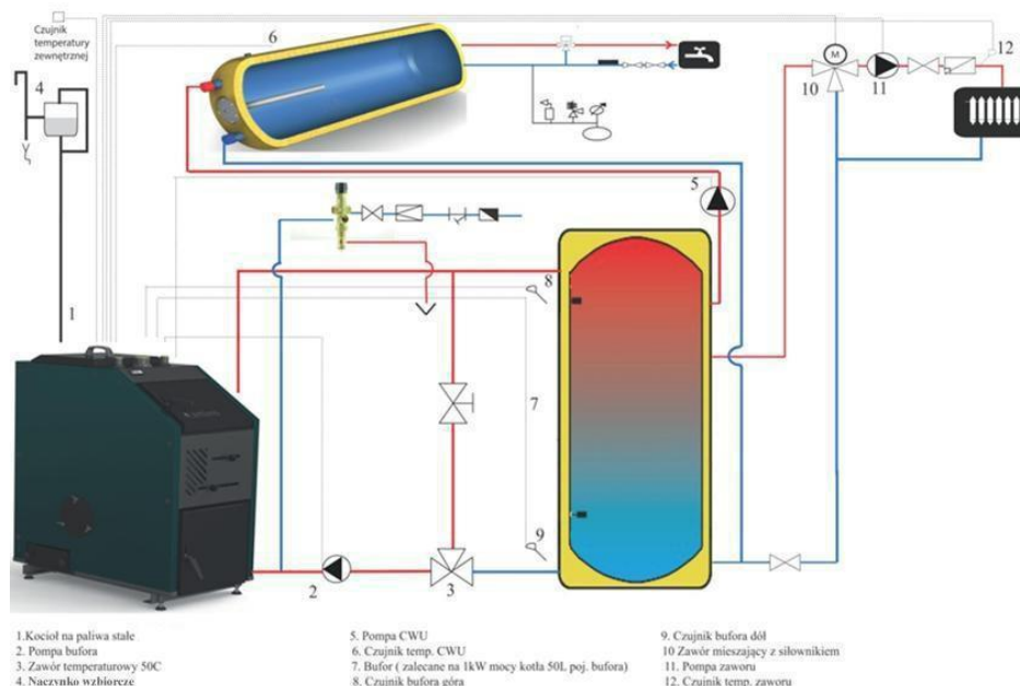
Rys. 5. Przykładowe schematy podłączeń kotła do instalacji grzewczej
